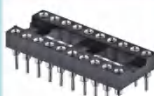
7210系列 2.54mm IC座 圆孔座 180度
