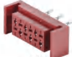
4000系列 红色IDC 母座有耳 180度
